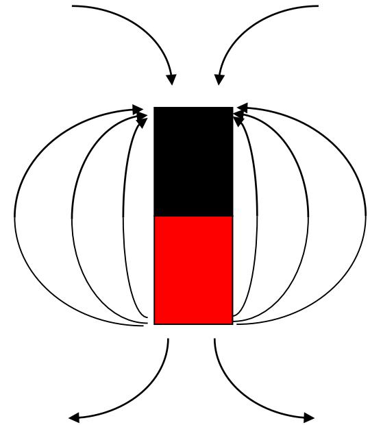
Magnetfeld
